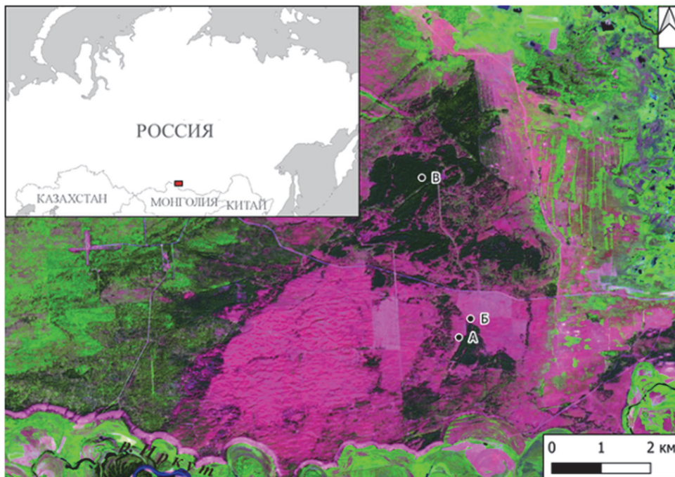
Рис. 1. Территория исследования на карте мелкого масштаба (карта-врезка) и на снимке Landsat 8 (август 2017 г., сочетание каналов 7-5-4). А, Б, В – площадки натурных наблюдений
