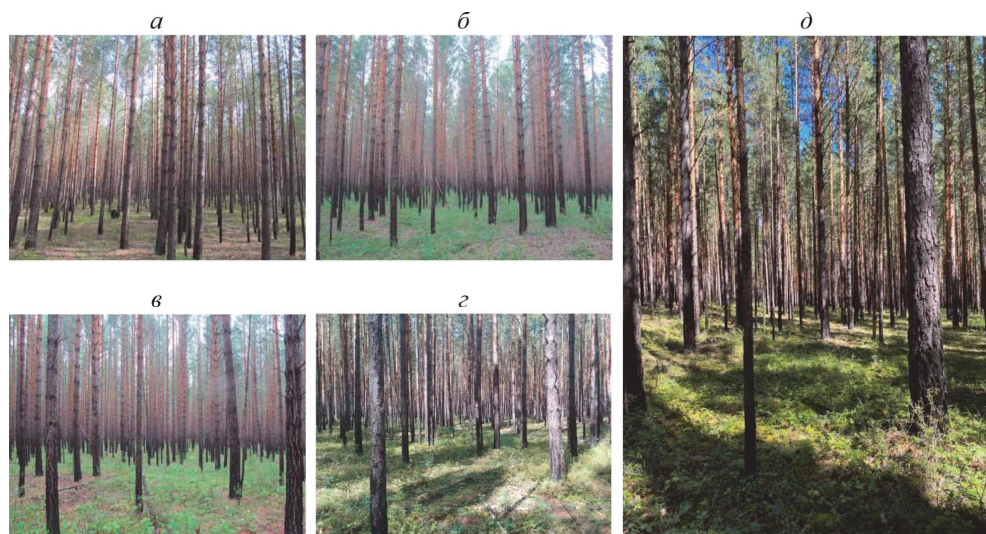
Рис. 3. Влияние проективного покрытия живого напочвенного покрова на показатели NBR фоновом участке в зависимости от фаз вегетации: а – начало вегетационного периода, проективное покрытие травяного покрова не превышает 30 % (05.06.2014, NBR = 0,550); середина вегетационного периода, проективное покрытие травостоя оценивается на уровне 70–80 %: б (25.07.2016, NBR = 0,650), в (08.08.2020, NBR = 0,638), г (03.08.2022, NBR = 0,685), д (12.08.2025, NBR = 0,713)
