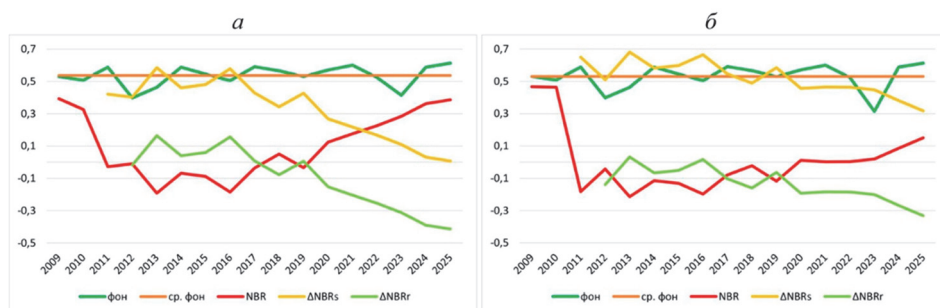
Рис. 4. Динамика показателей NBR и dNBR начала вегетационного периода в 2009–2025 гг. на ключевых участках урочища Бадары: а – гарь сильной степени огневого поражения (площадка А), б – гарь очень сильной степени огневого поражения (площадка Б)
